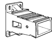
DM300 Mensola di sostegno. Bracket. 80x200x150 mm
