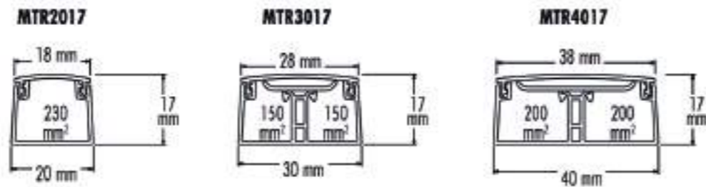
Sezione utile e capacità di contenenza cavi H07V - U/R/K Wire fill capacity H07V - U/R/K
